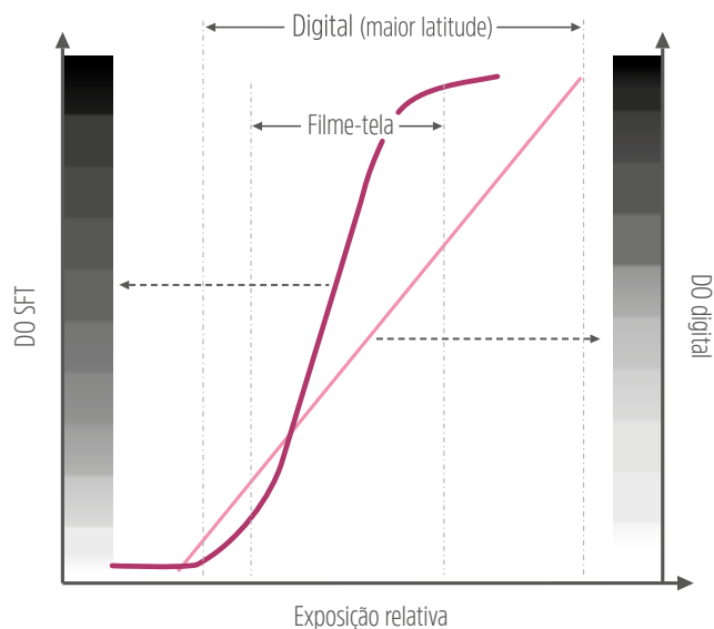
Figura 30. Resposta da combinação SFT intensificadora (à esquerda, curva senoidal) em comparação com a resposta do detector digital (à direita, linear, reta)
