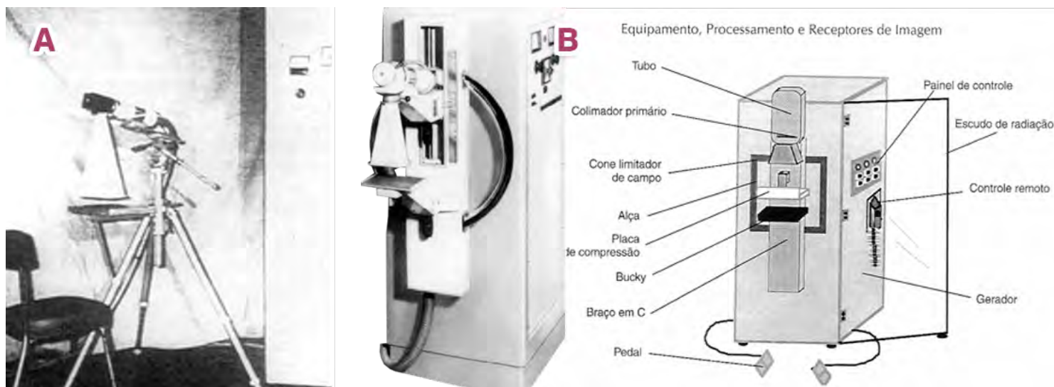
Figura 18. (A) Primeiro mamógrafo. Protótipo de 1965 chamado de Treipied. (B) Primeiro modelo comercial do Senographe, lançado em 1966
