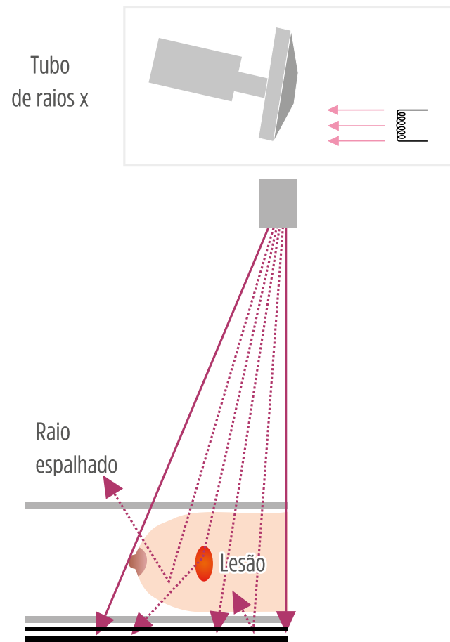
Figura 19. Processo de produção da imagem na mamografia
