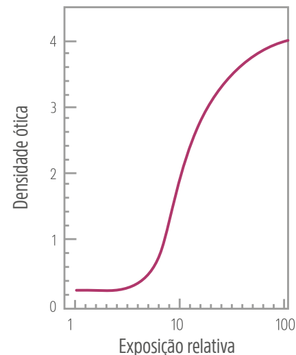
Figura 28. Curva característica do filme para o sistema tela-filme
