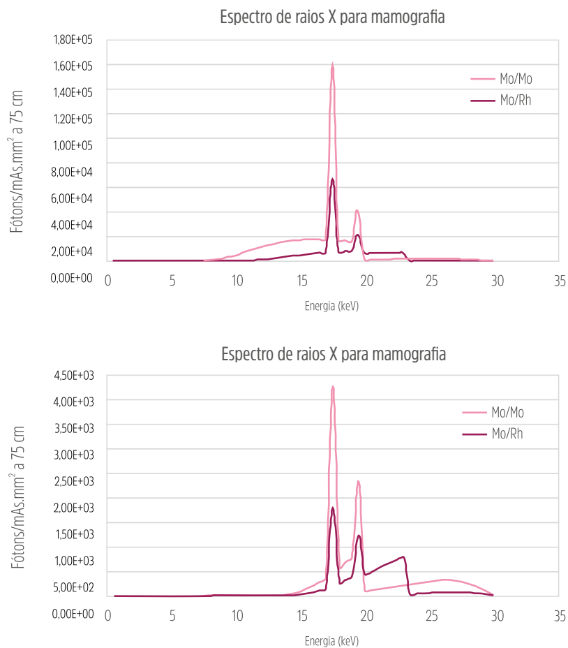
Figura 25. Espectros de raios X para duas combinações alvo-filtro
