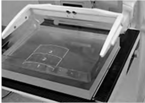
Figura 91. Bloco de acrílico posicionado no mamógrafo para o teste
