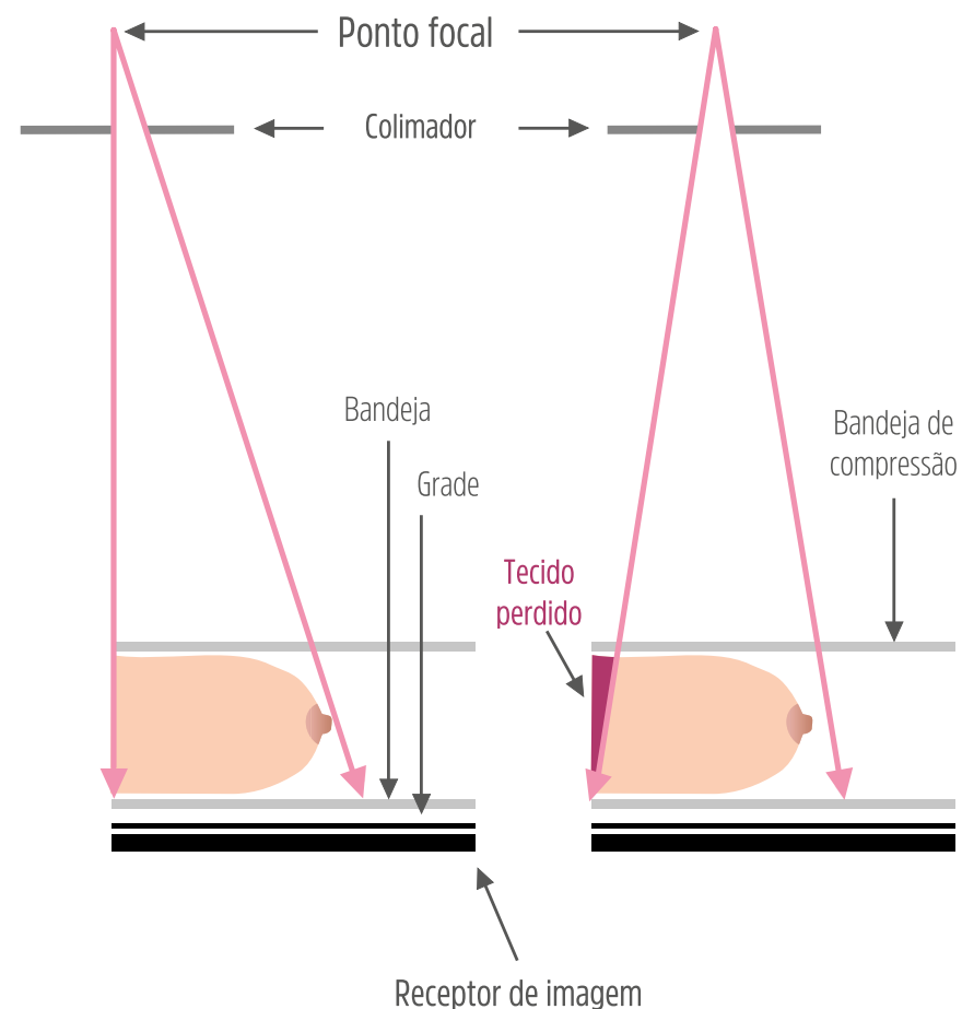
Figura 23. Geometria básica do feixe de raios X
