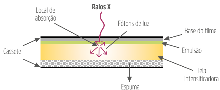
Figura 27. Processo de absorção dos raios X
