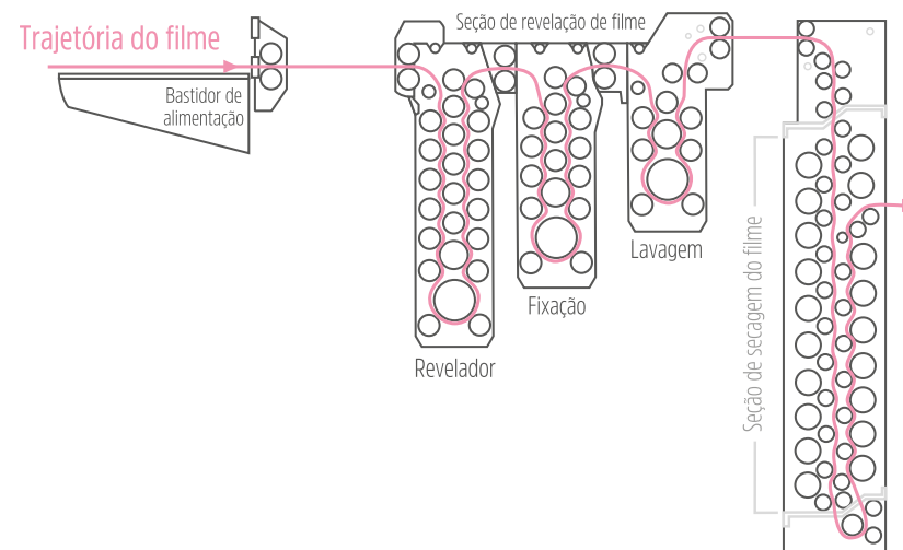
Figura 32. Etapas do processamento do filme radiográfico
