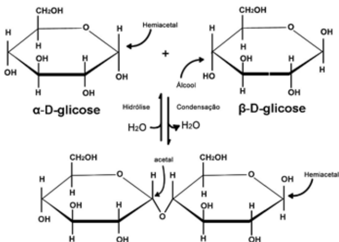
Figura 1.14. Formação da ligação glicosídica na síntese da maltose.
