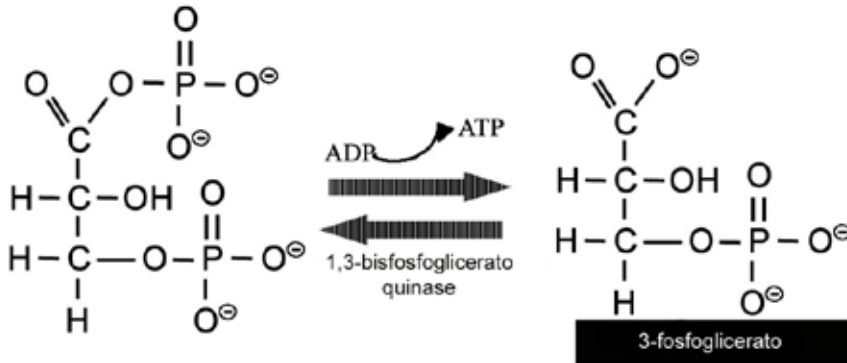
Figura 1.27. Primeira reação com produção de ATP.
