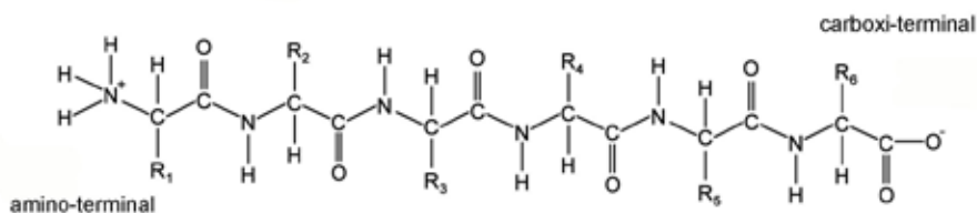
Figura 1.5. Estrutura primária de uma proteína.
