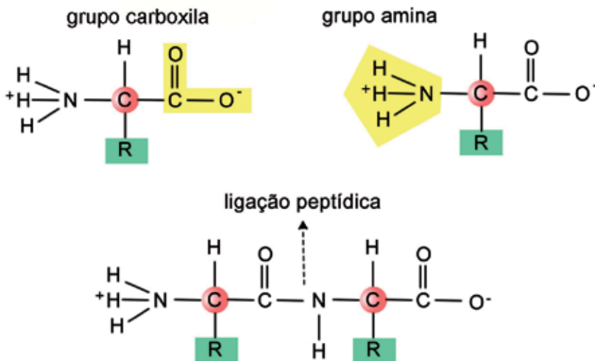
Figura 1.4. Ligação peptídica.
