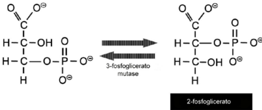
Figura 1.28. Formação do 2-fosfoglicerato.
