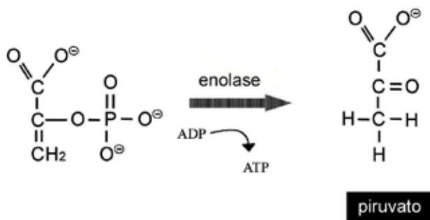
Figura 1.30. Formação do piruvato e de ATP.
