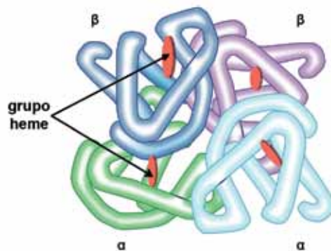
Figura 1.8. Estrutura quaternária da hemoglobina mostrando os grupos hemes.
