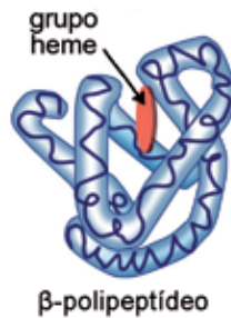
Figura 1.7. Estrutura terciária da cadeia de globina mostrando grupamento heme.
