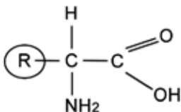
Figura 1.2. Fórmula geral de um aminoácido.
