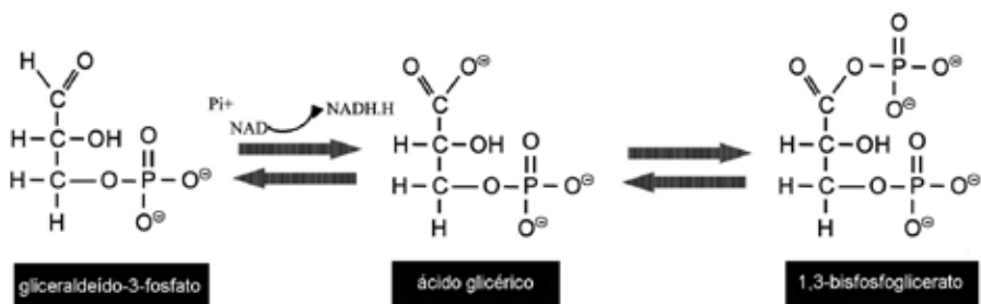
Figura 1.26. Formação do 1,3-bisfosfoglicerato.
