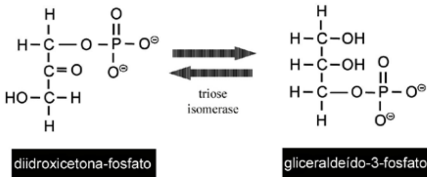
Figura 1.25. Isomerização da diidroxicetona-fosfato ao gliceraldeído-3-fosfato.
