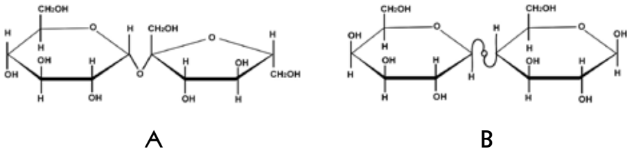
Figura 1.13. A) Estrutura da sacarose; B) Estrutura da lactose.
