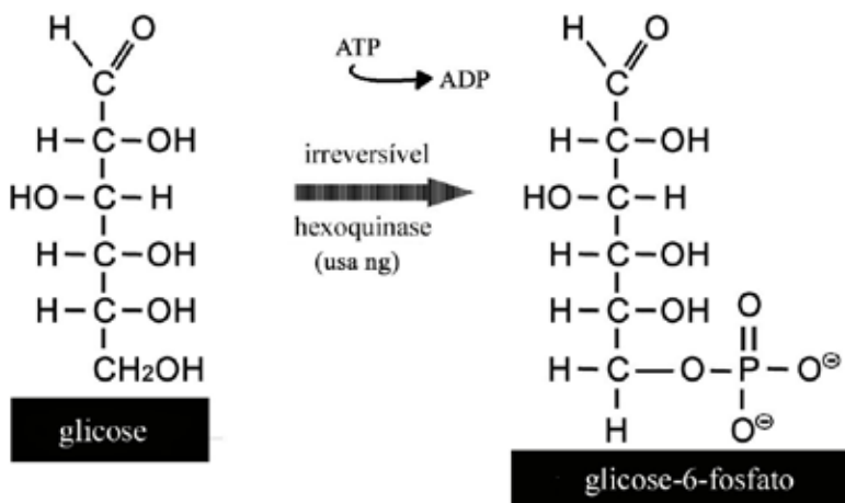
Figura 1.23. Fosforilação da glicose pela hexoquinase.
