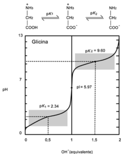
Figura 1.3. Curva de titulação da glicina.
