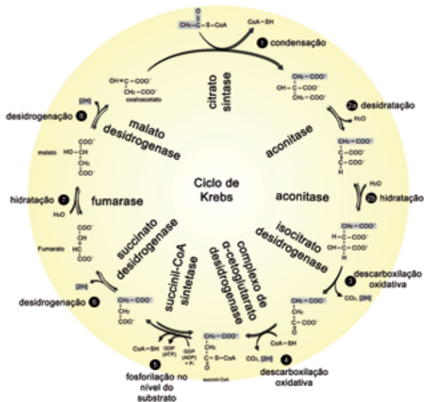
Figura 1.34. Reações do ciclo de Krebs.
