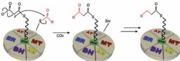
Figura 1.36. Ciclo de biossíntese de um ácido graxo.
