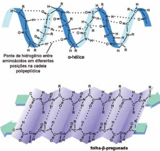
Figura 1.6. Estruturas secundárias organizadas das proteínas.
