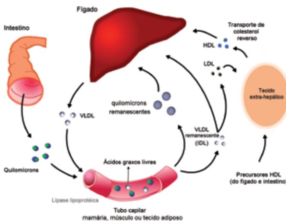
Figura 1.20. Lipoproteínas e transporte de lipídios.
