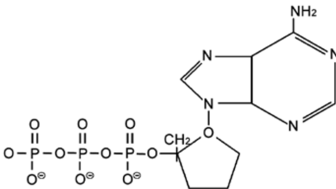
Figura 1.21. Molécula de ATP.
