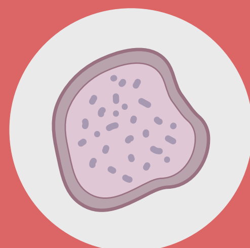
Célula normal
