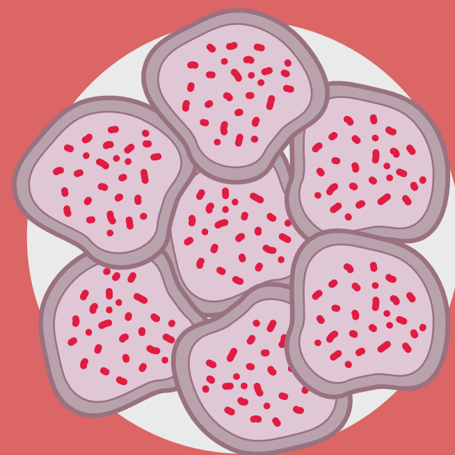
Célula cancerosa
